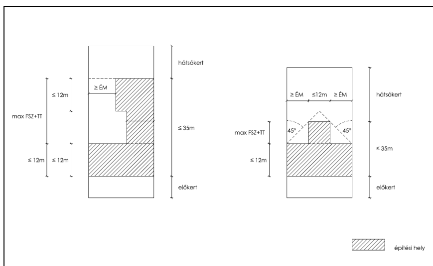
Zárt sorú beépítési mód beépítési lehetőségei (magyarázó ábra)
