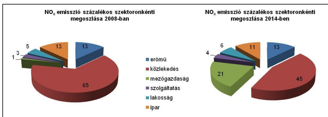
5. ábra NO x emisszió megoszlása szektoronként 2008. és 2014. évben
