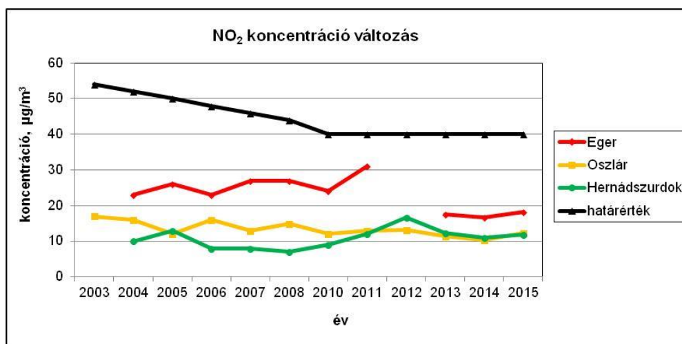
4. ábra A NO 2 koncentráció változása az Egerben üzemelő mérőállomáson
