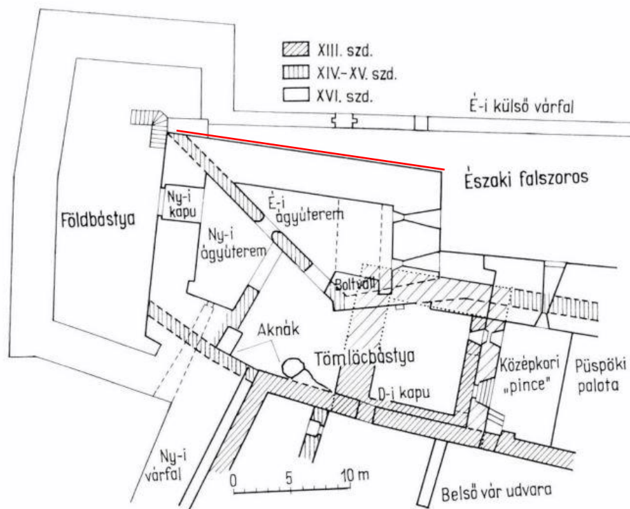
247. kép. A Tömlőcbástya alaprajza
