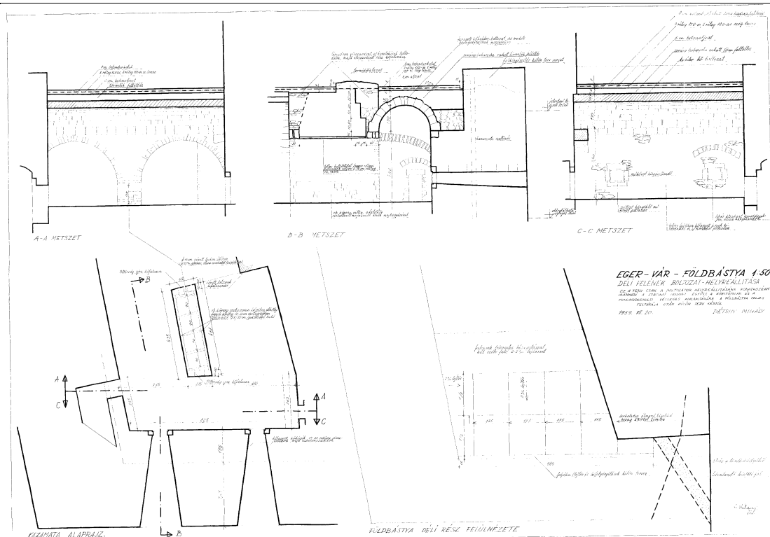
A Földbástya déli fele boltozatának helyreállítási tervei Détsy Mihály 1959 MÉM-MDK Tervtár 1338
