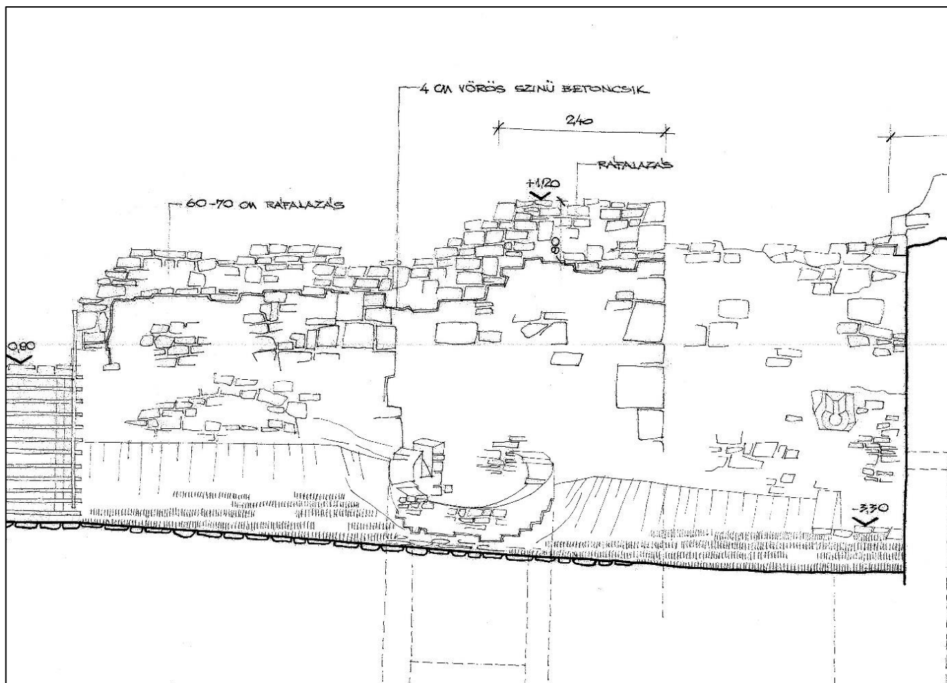
Sedlmayr János helyreállítási terve (részlet), 1963. MÉM-MDK Tervtár 14811
