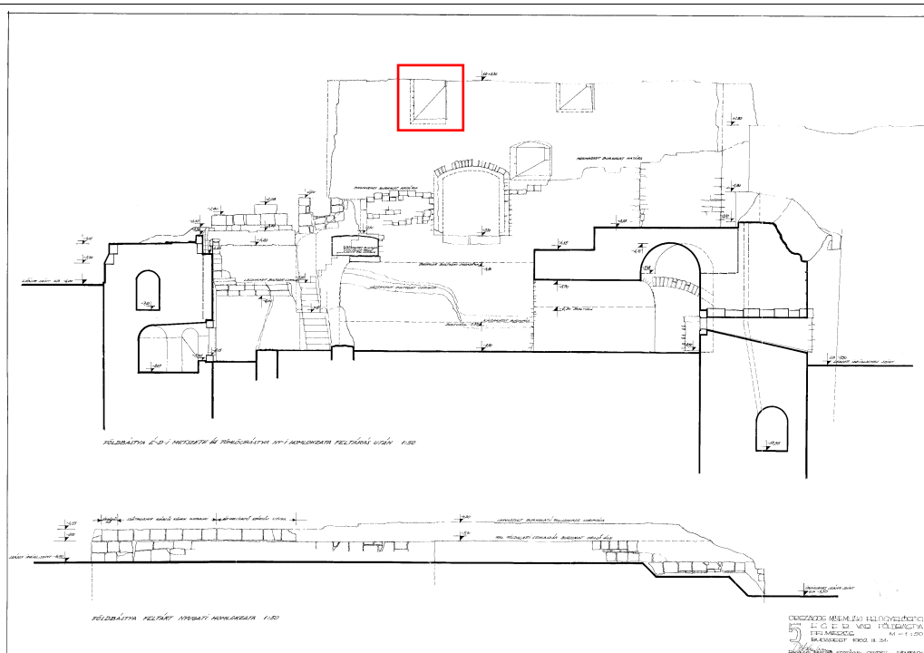
Tömlőcbástya és Földbástya nyugat felől, felmérés, Détsy Mihály, 1962. MÉM-MDK Tervtár 15271
