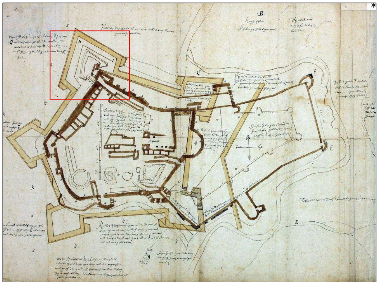
Ottavio Baldigara „C” terve, lent ennek részlete a bástyákkal
