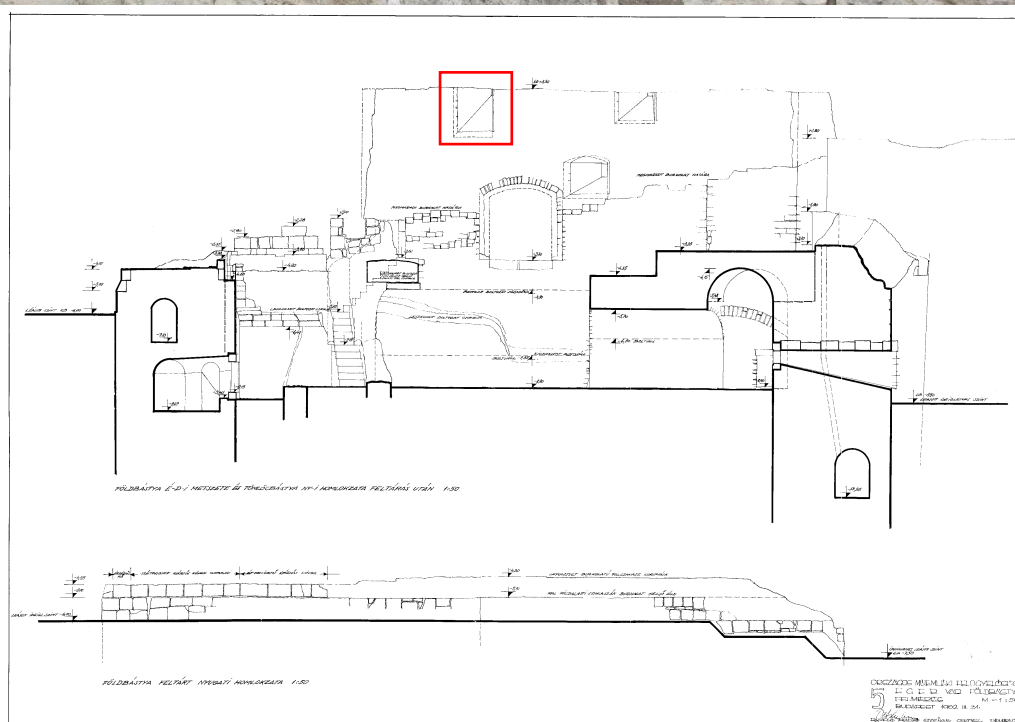
Tömlöcbástya és Földbástya nyugat felől, felmérés, Détsy Mihály, 1962. MÉM-MDK Tervtár 15271
