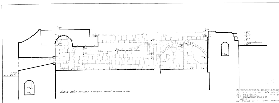
Eger, vár, a Földbástya felmérése Détsy Mihály 1962. MÉM-MDK Tervtár 15270
