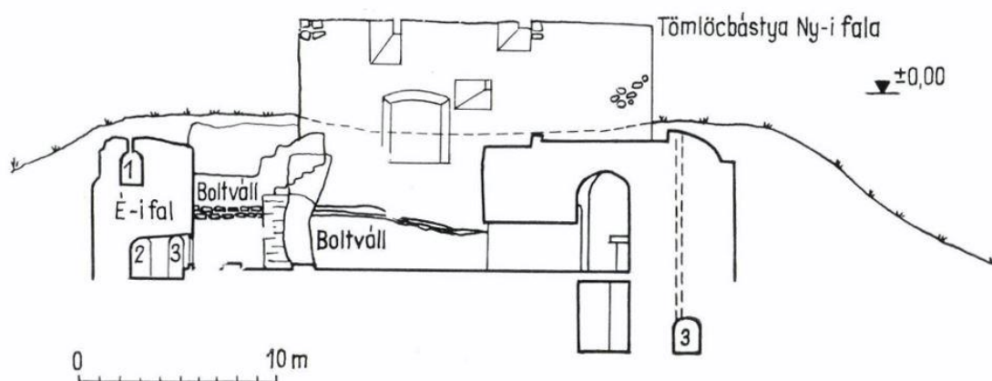
275. kép. A Földbástya észak—déli metszete
