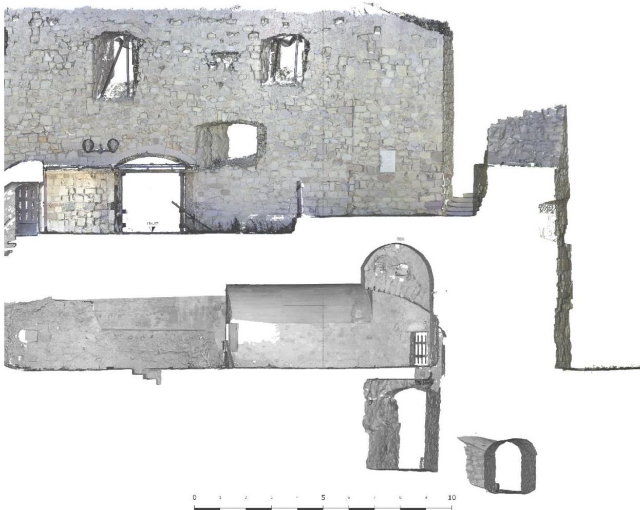
Tömlöcbástya nyugati homlokzat, digitális felmérés, MindiGIS Kft, 2025
