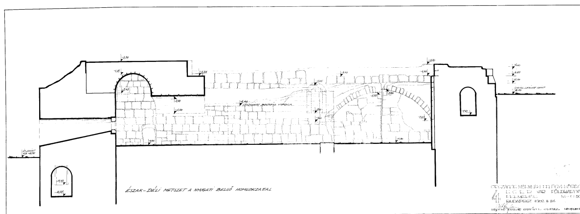
A FÖLDBÁSTYA északi termének metszete a feltárás után, Détsy Mihály 1962, MÉM-MDK Tervtár 15269. lent az észak-déli belső metszet, 15270
