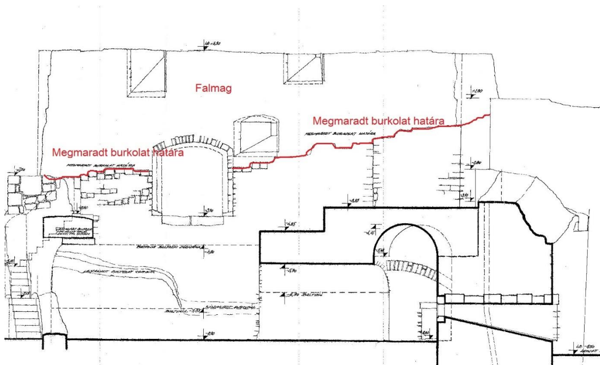
Tömlőcbástya és Földbástya nyugat felől, felmérés és helyreállítási koncepció, Détsy Mihály, 1962. MÉM-MDK Tervtár 15271, lent: Sedlmayr János, Nándori Klára 1963. 27470
