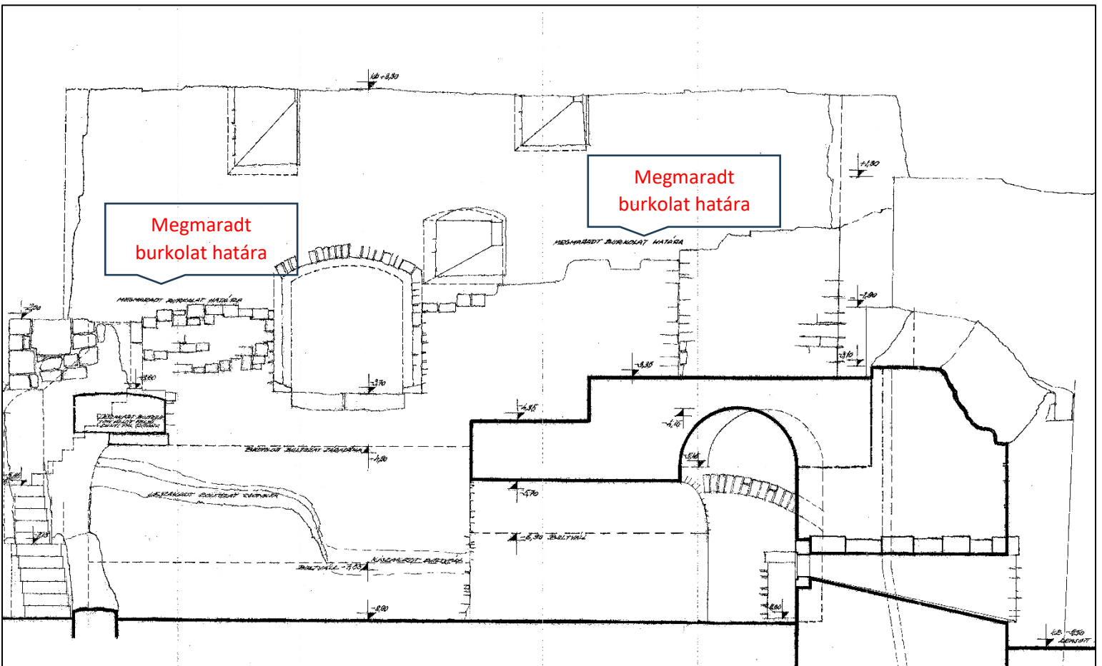
TÖMLÖCBÁSTYA ÉS FÖLDBÁSTYA NYUGAT FELŐL, FELMÉRÉS ÉS HELYREÁLLÍTÁSI KONCEPCIÓ, DÉTSY MIHÁLY, 1962. MÉM-MDK TERVTÁR 15271, LENT: SEDLMAYR JÁNOS, NÁNDORI KLÁRA 1963. 27470 A MEGMARADT EREDETI FALKORONA ÉS FALBURKOLAT JELÖLÉSÉVEL.
