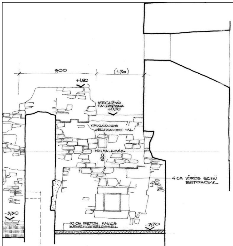
Sedlmayr János helyreállítási terve (részlet), 1963. MÉM-MDK Tervtár 14811
