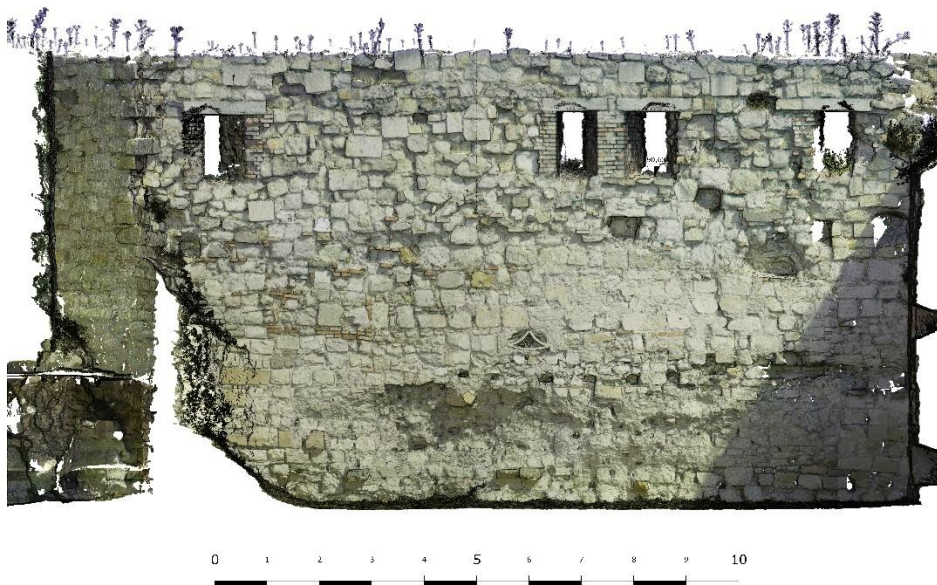
Tömlöcbástya, északi fal belső, digitális felmérés, MindiGIS Kft , 2025
