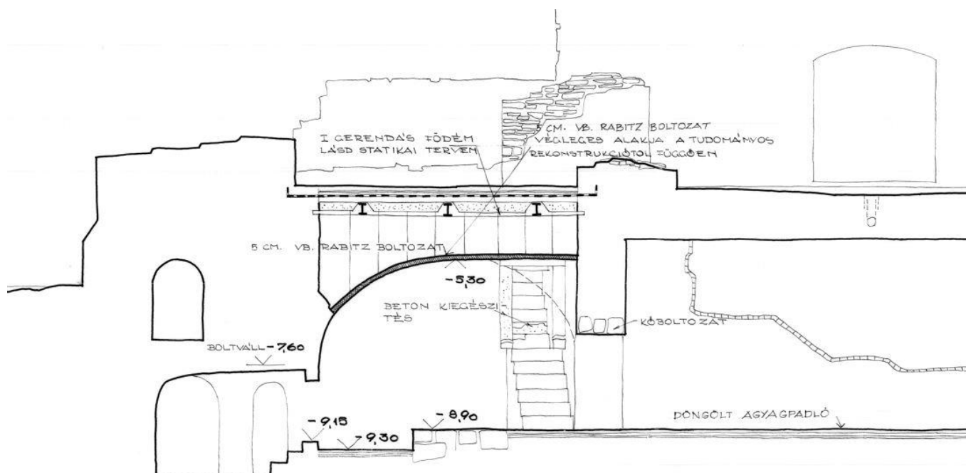
B-B METSZET M = 1:50
