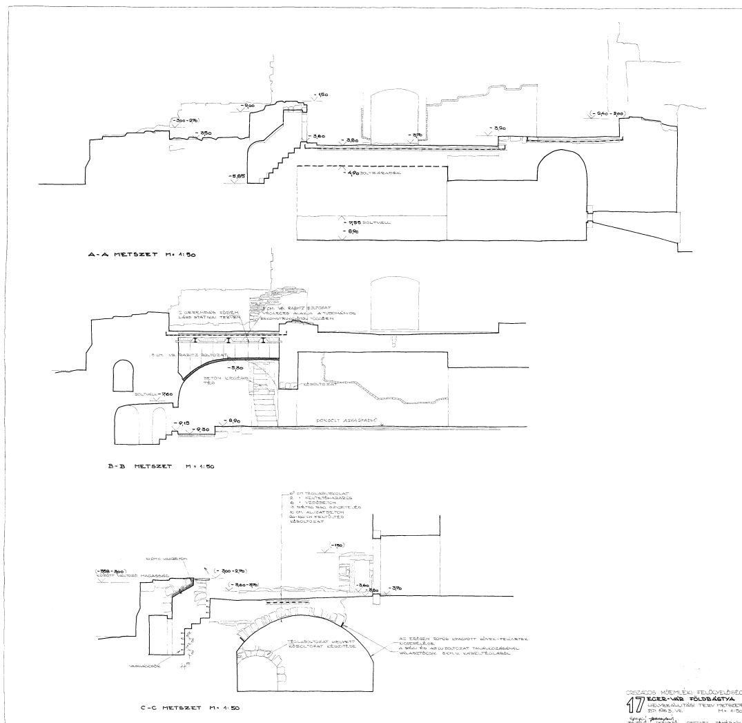
Földbástya, helyreállítási terv, metszetek Sedlmayr János, 1963. MÉM-MDK Tervtár 13526
