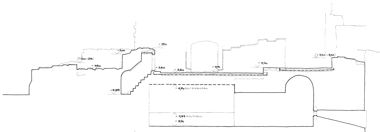
A-A METSZET M = 1:50
