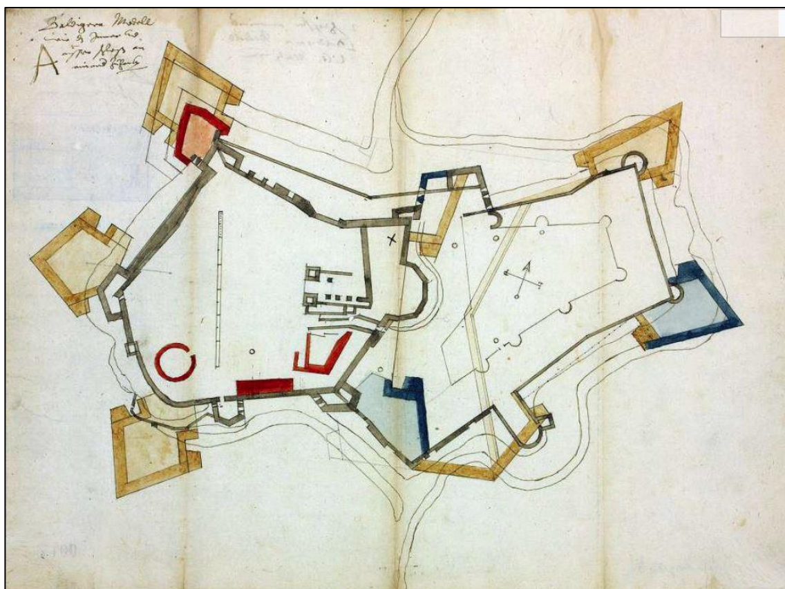
Ottavio Baldigara „A” terve 1572
