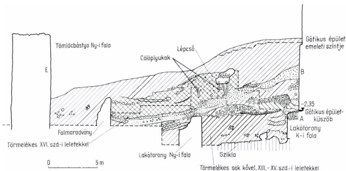
248. kép. A bástya nyugat—keleti metszete
