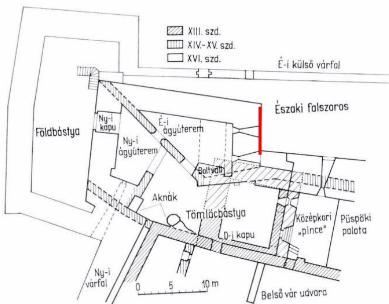
247. kép. A Tömlőbástya alaprajza
