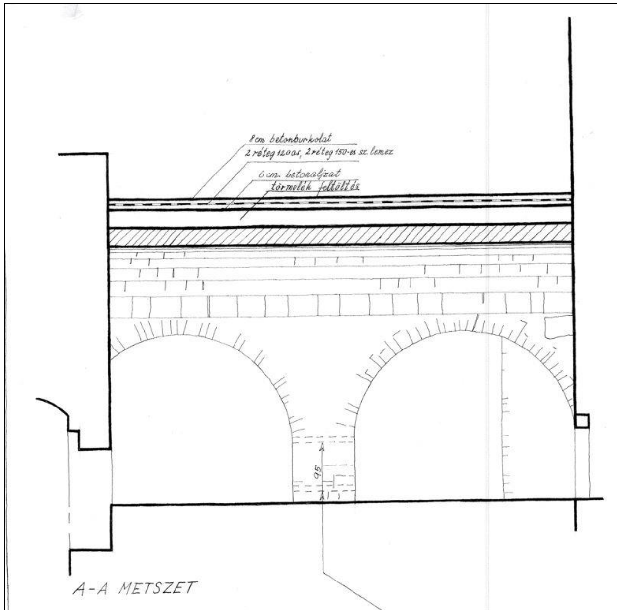
A födém helyreállítása (A déli ágyúterem boltozatának helyreállítása, részlet), Détsy Mihály 1959 MÉM-MDK 1338
