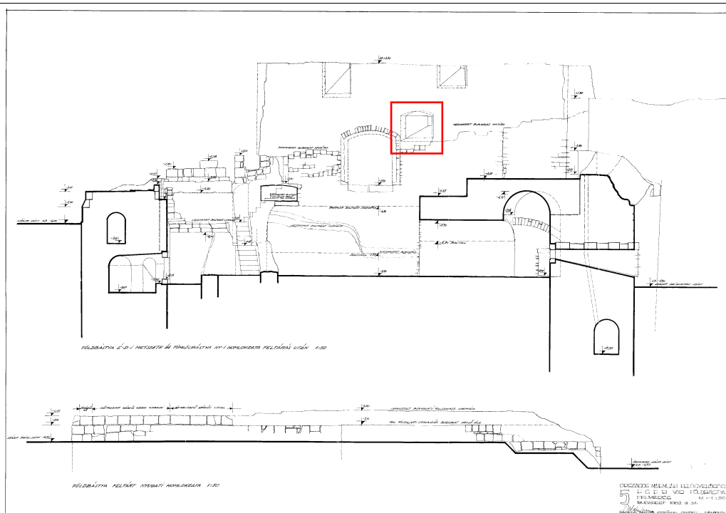
Tömlőcbástya és Földbástya nyugat felől, felmérés, Sedlmayr János, 1962. MÉM-MDK Tervtár 15271
