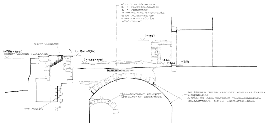
C-C METSZET M = 1:50
